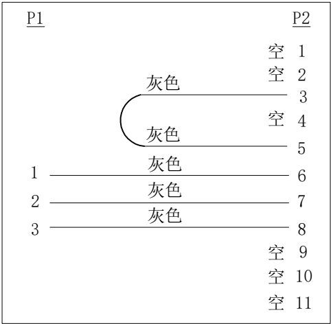
接 线 图
