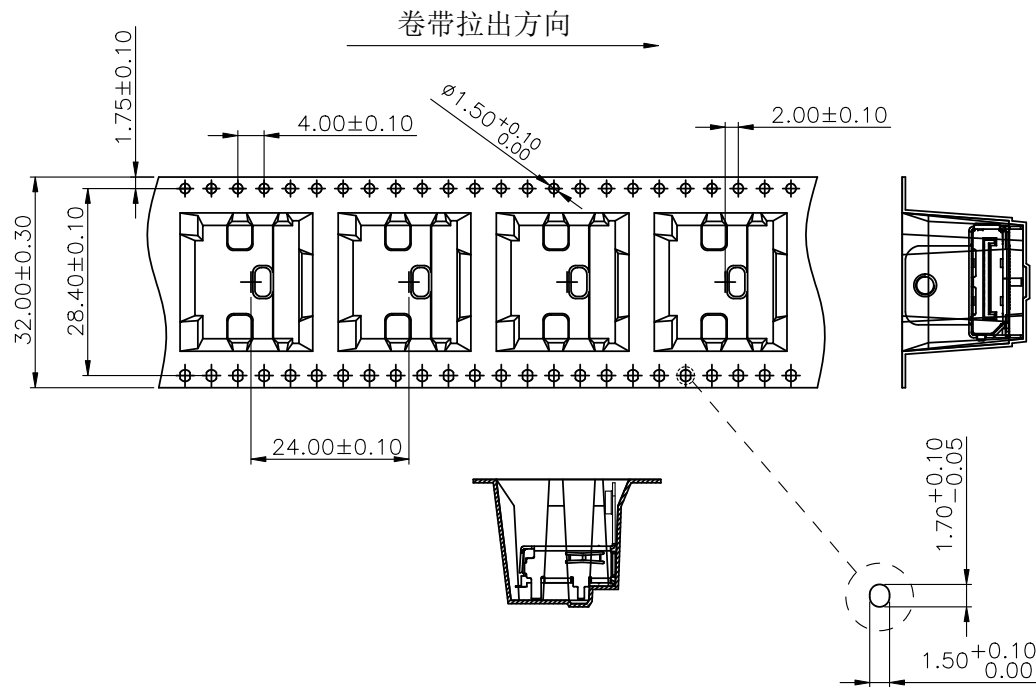
DETIAL A 2:1
